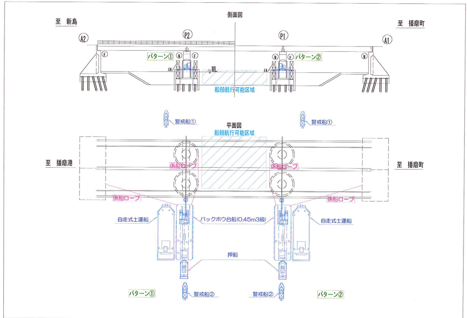
播磨大橋 施工状況図
