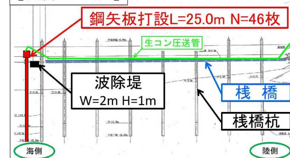
【西宮BP工区】 縦断面図
