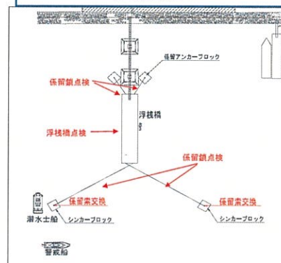
作業状況図
